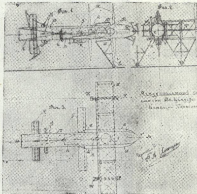
Самолет-ракета системы Цандера
